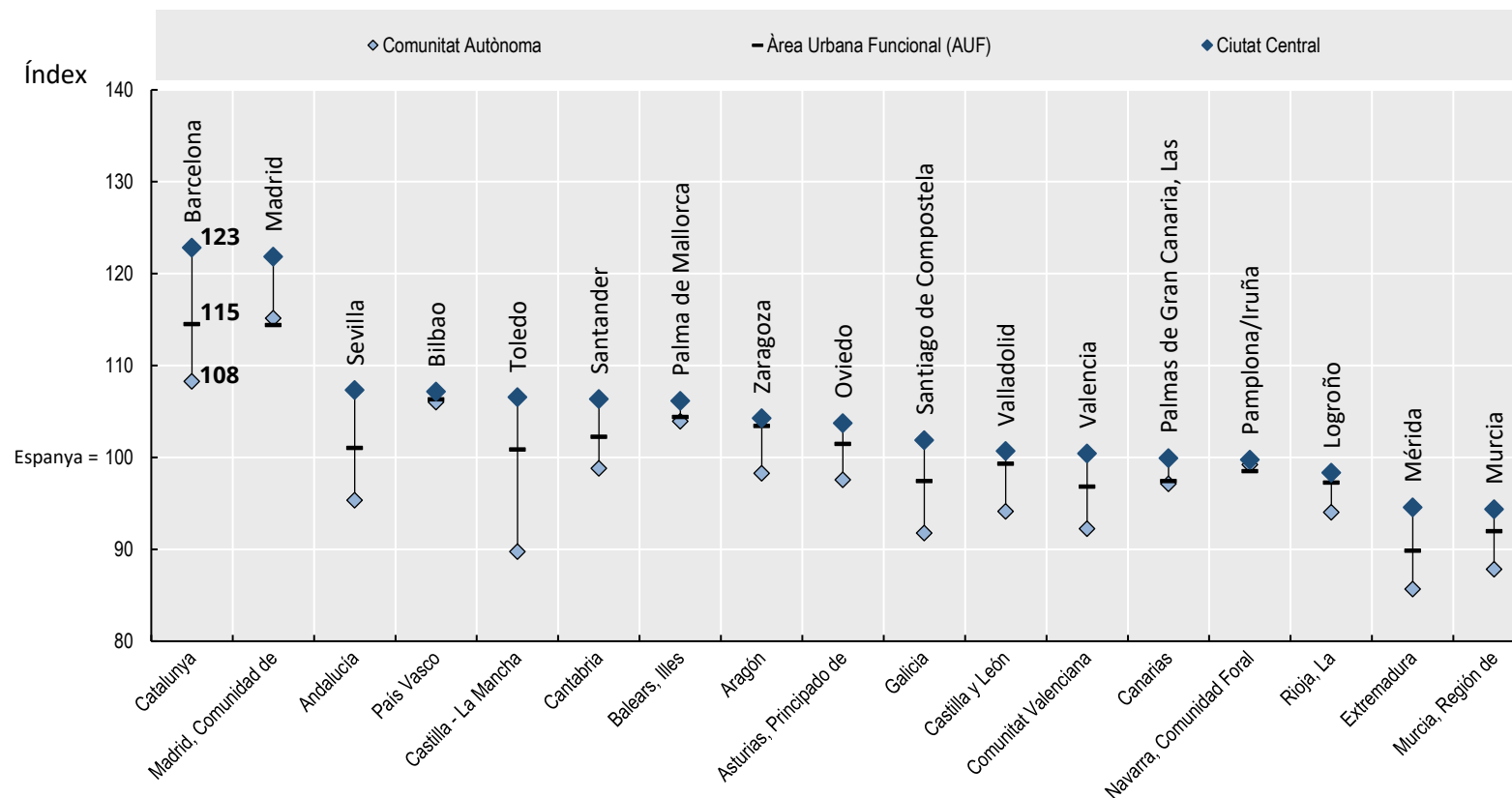
PPA de les CCAA, Àrees Urbanes Funcionals i les ciutats centrals, 2018
